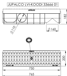
Tarvitavat poistot tehdään esim. reikäsaahalla. Yleiskuva malleille: PP100, PP200 ja PP250
