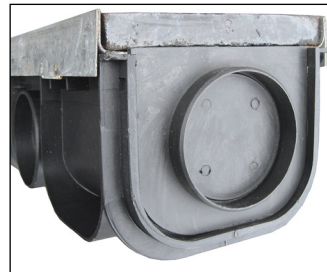
Päätäkappale yhdevarauksella. Yleiskuva malleille: PP100, PP200 ja PP250.
