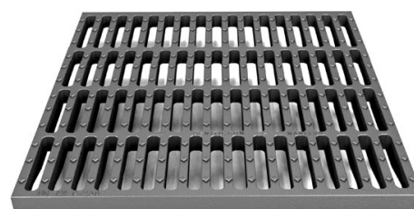
Sadevesikansi C250 750 x 600 x 27 mm
