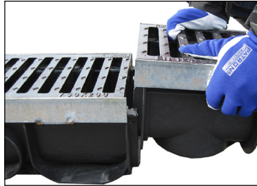
Helposti asennettava ponttikiinnitys.
